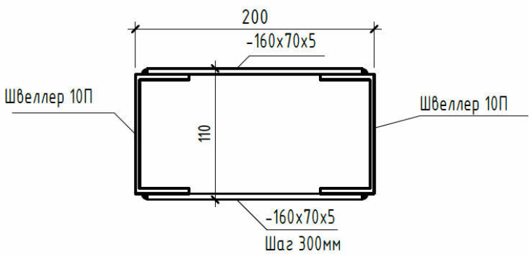
Узел 1 (1 : 5)
