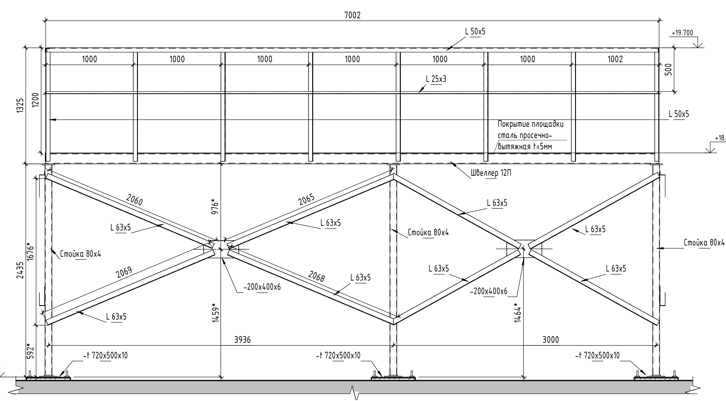
Вид 2 (1 : 20)
