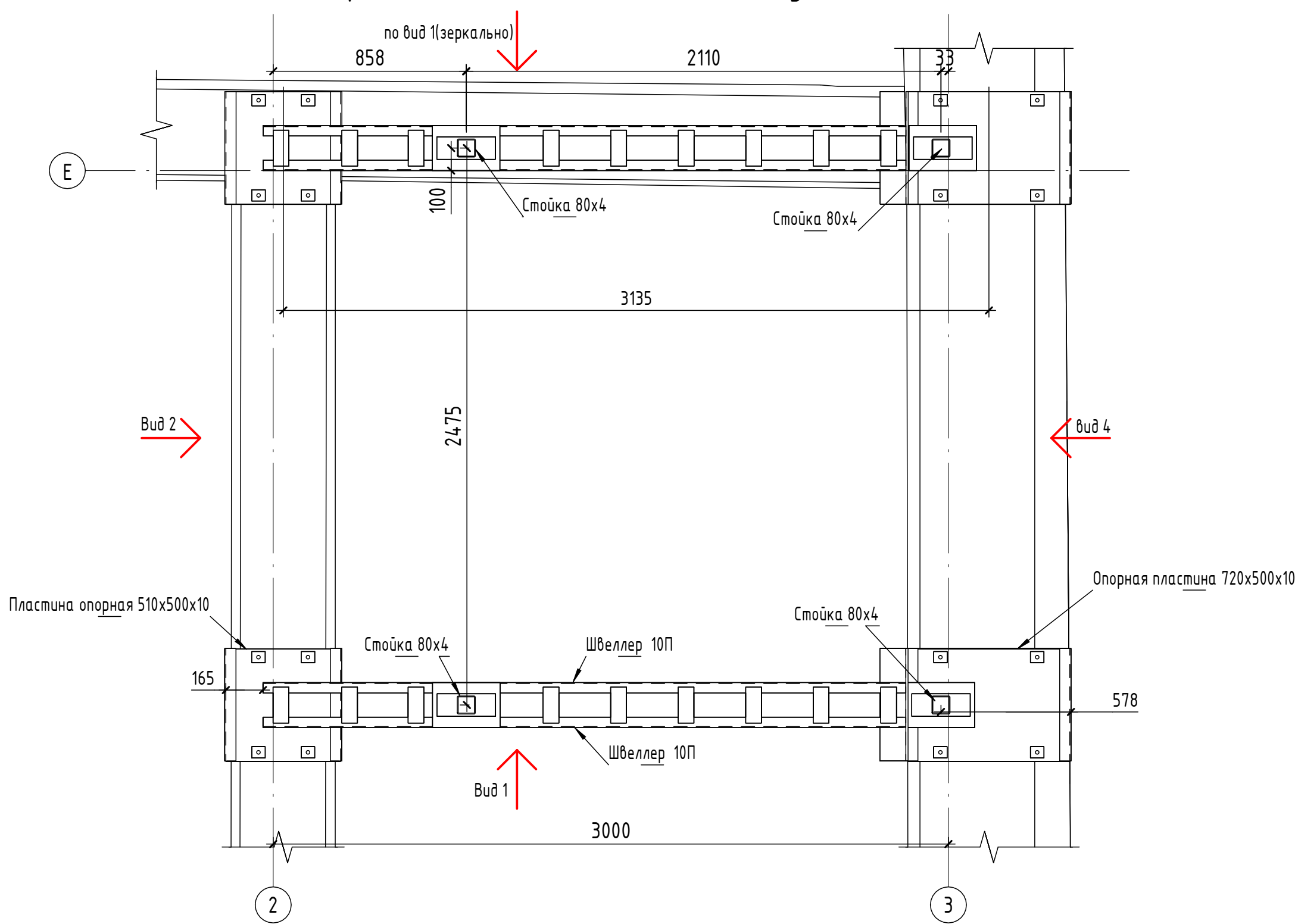
План опорных пластин и стоек под площадку Пл-1 (1 : 20)
