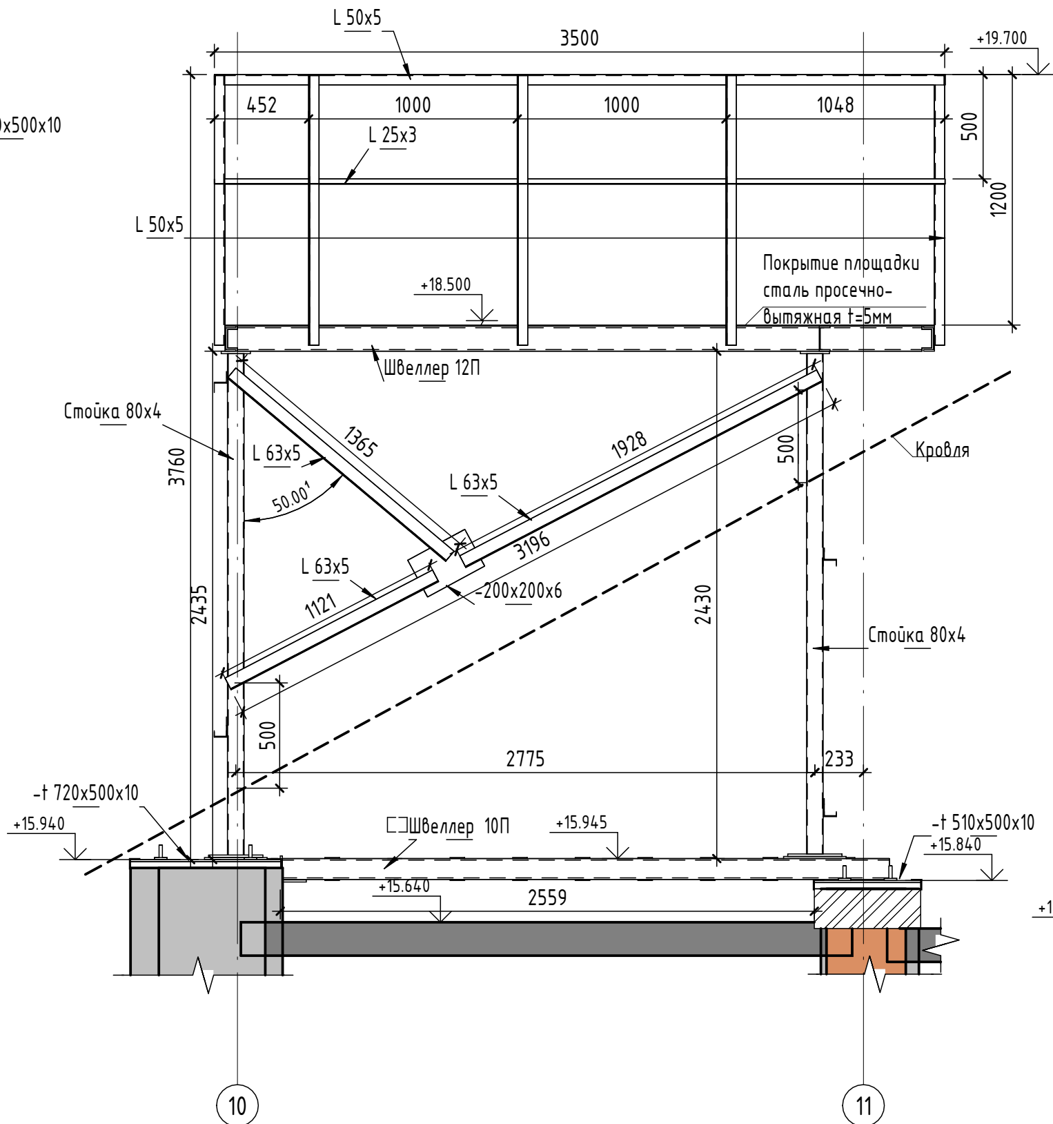
Вид 1 (1 : 20)
