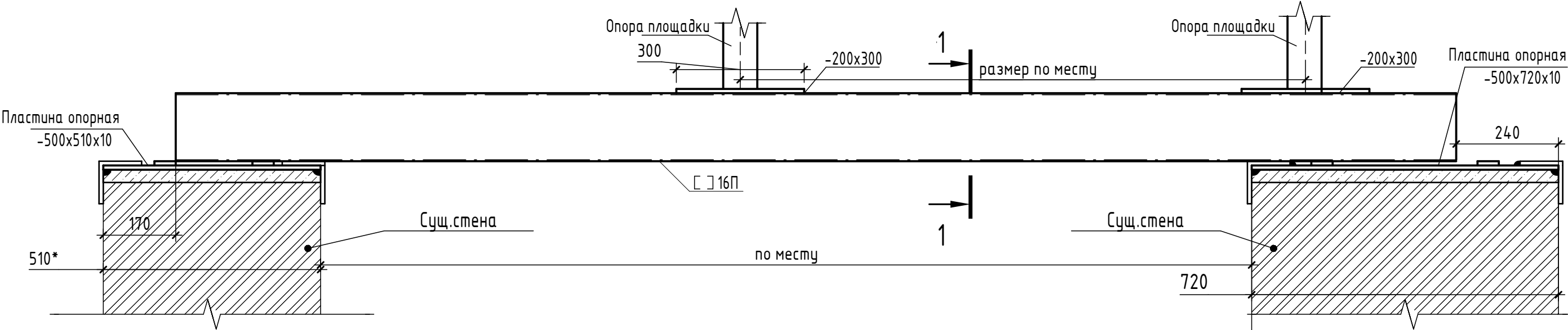
1-1.. ( 1 : 5)
