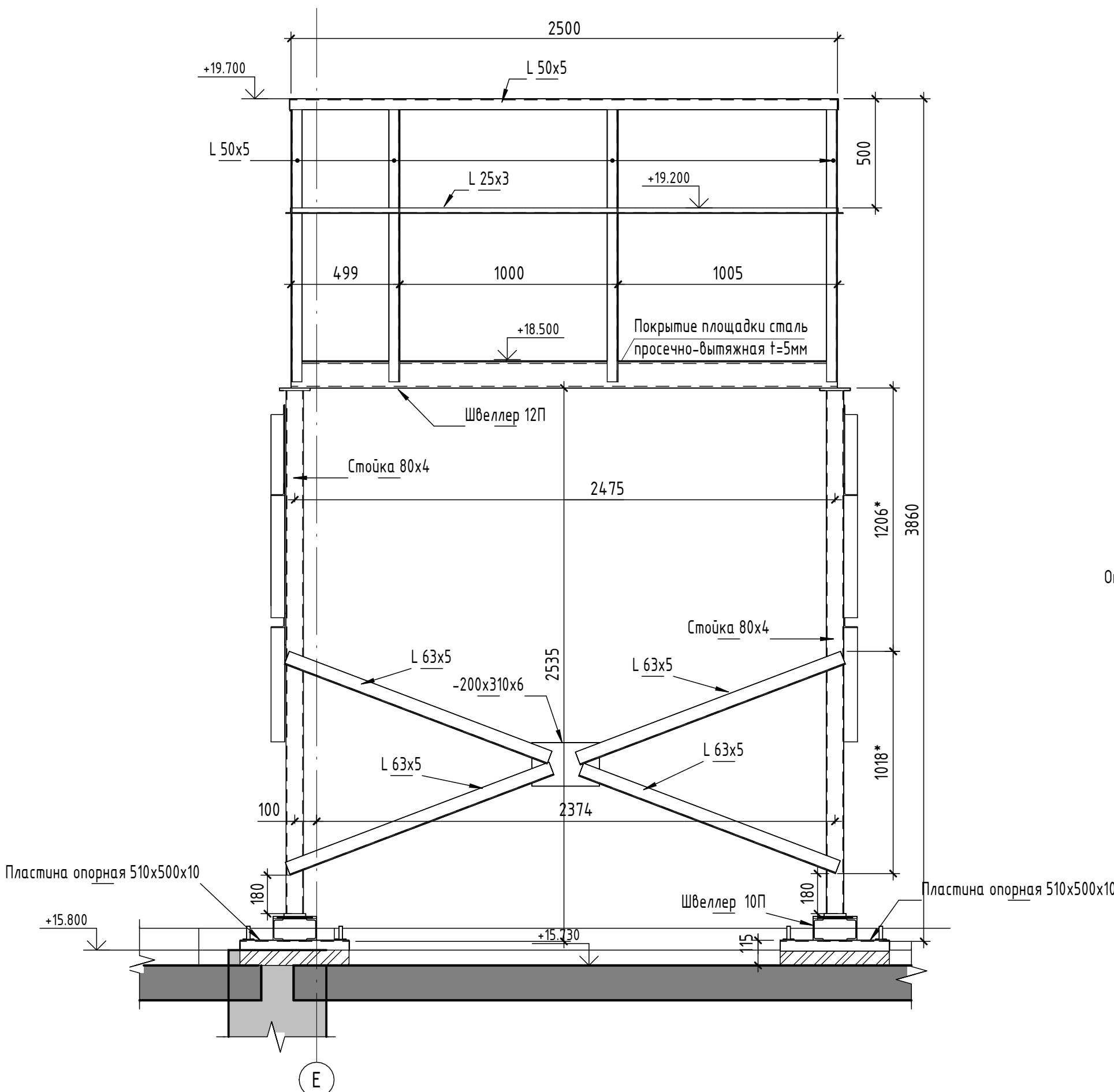
Вид 2 (1 : 20)
