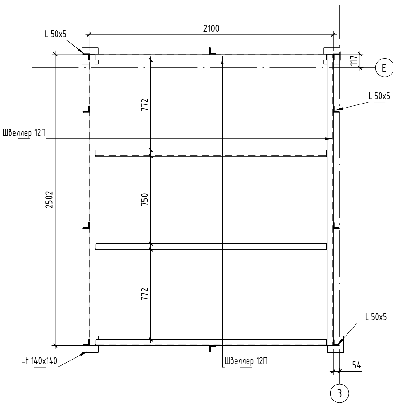
Вид 3(Площадка под настил) (1 : 20)
