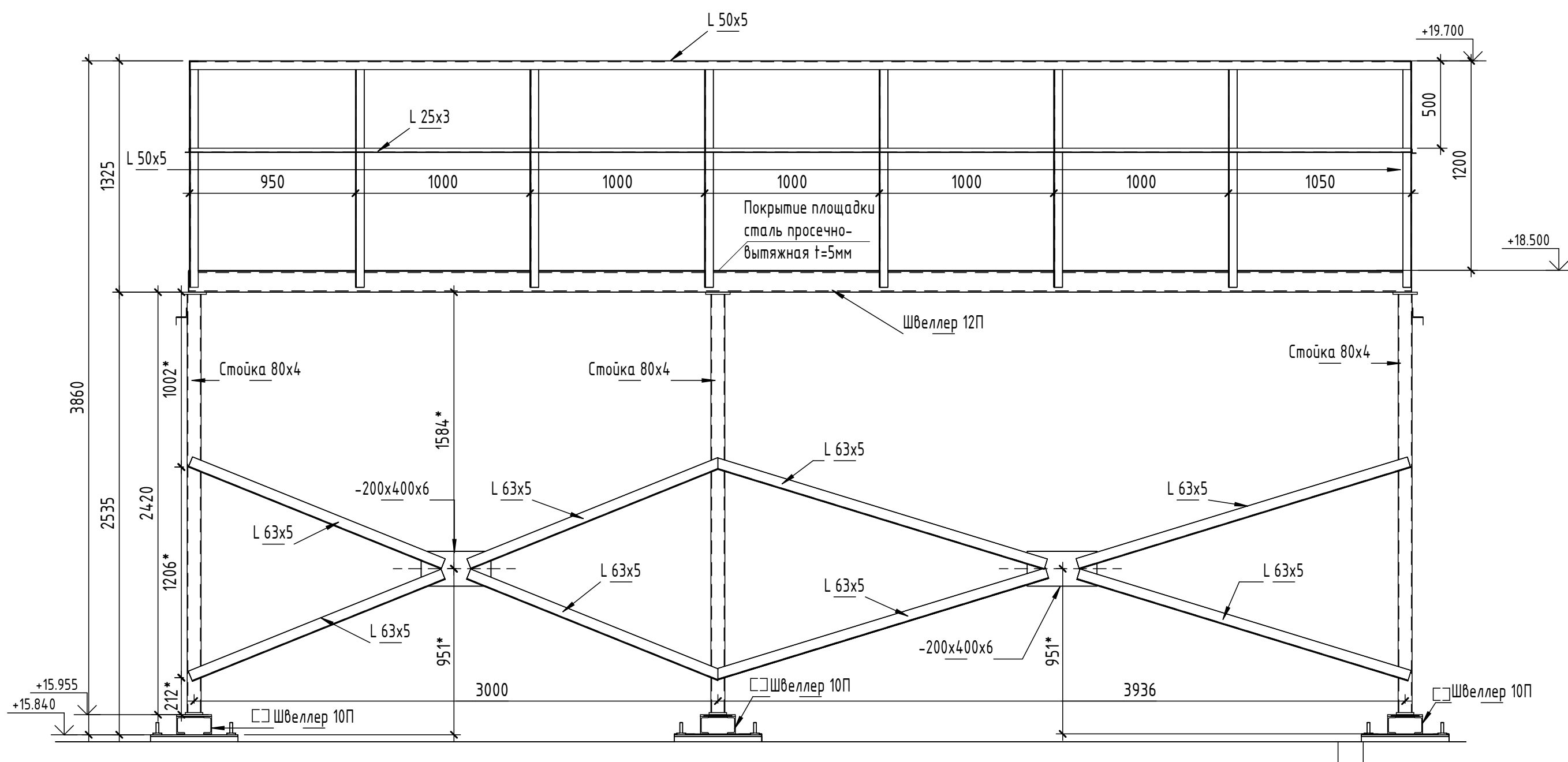
Вид 3 (1 : 20)
