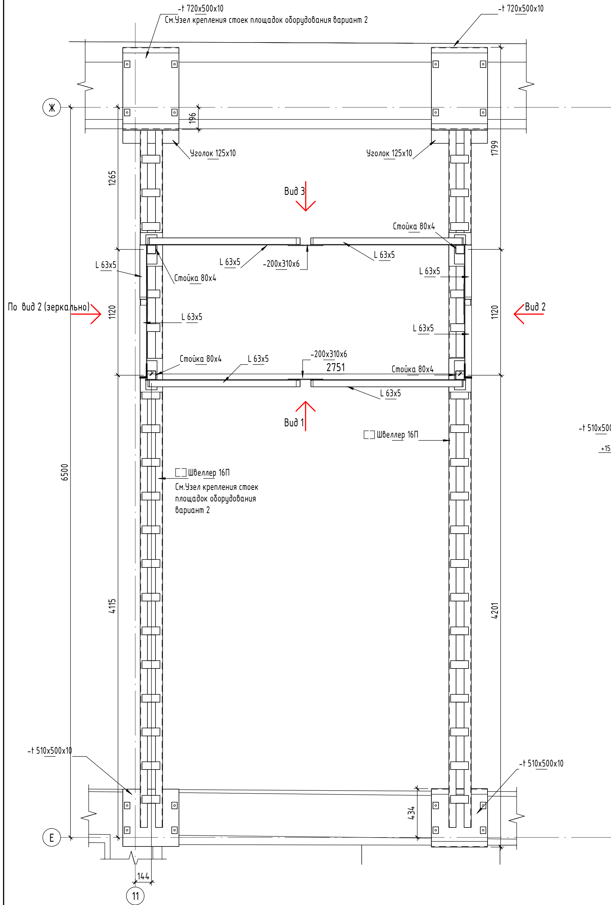
План опорных пластин и стоек под площадку Пл-9 ( 1 : 20)
