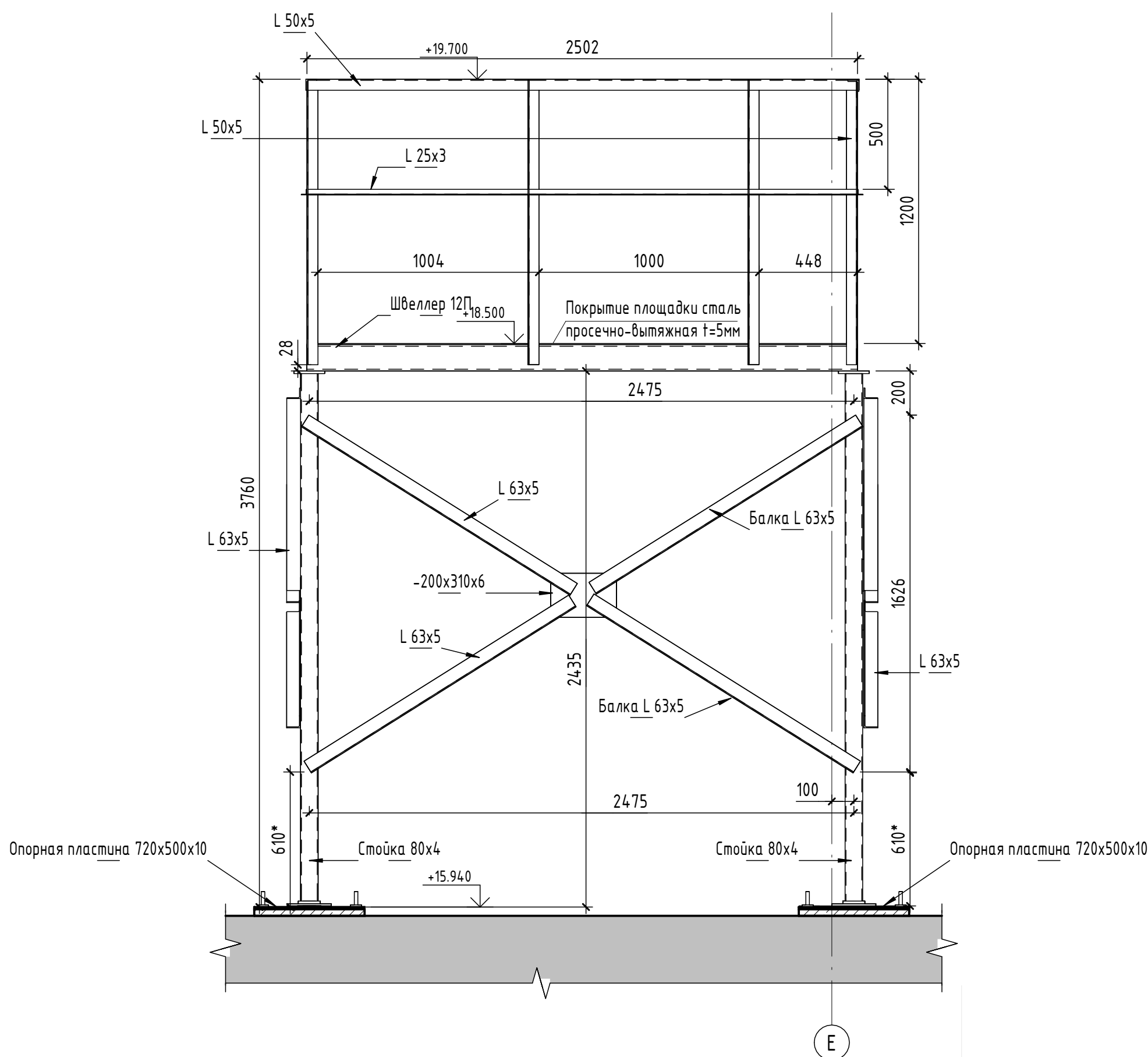
Вид 4 (1 : 20)
