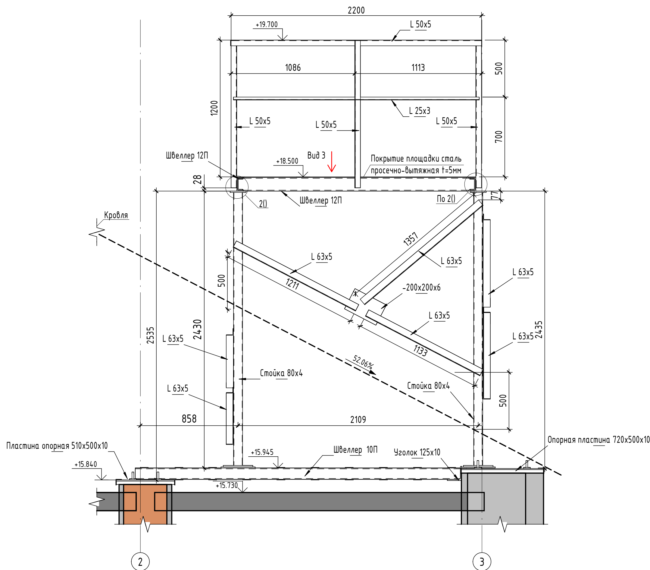
Вид 1 (1 : 20)
