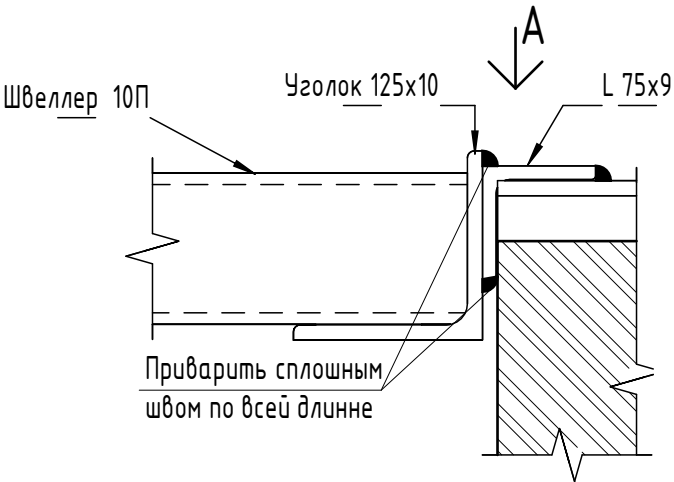
Узел 1 (1 : 5)
