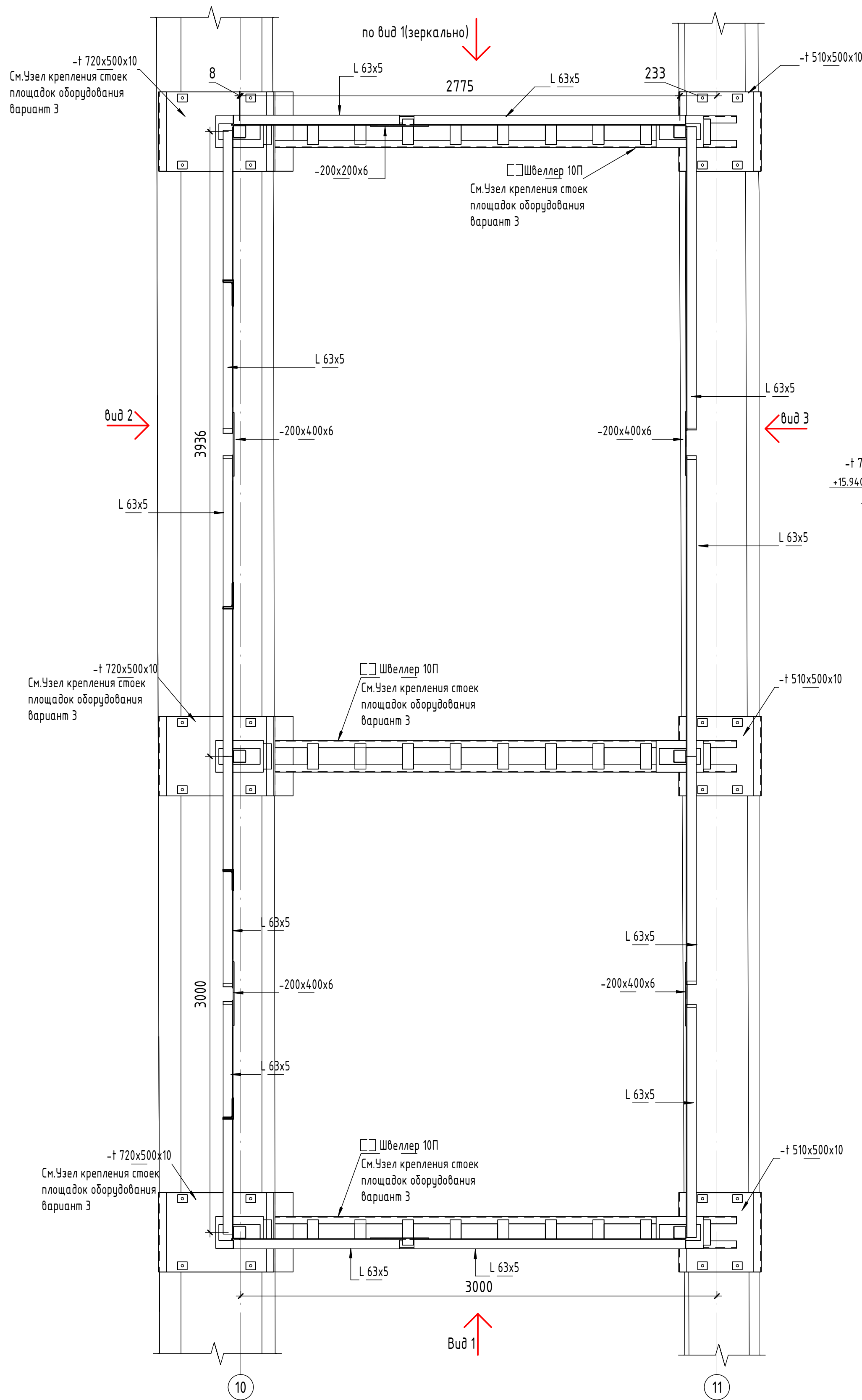
План опорных пластин и стоек под площадку Пл-7 (1 : 20)
