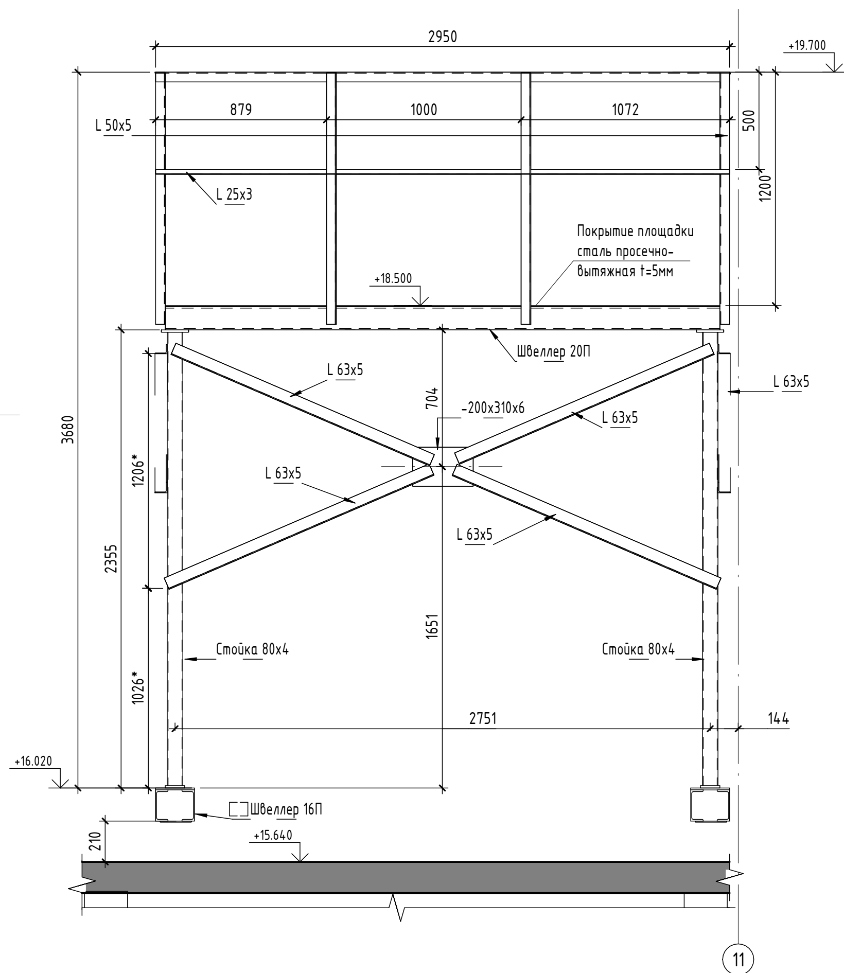
Вид 3 ( 1 : 20)
