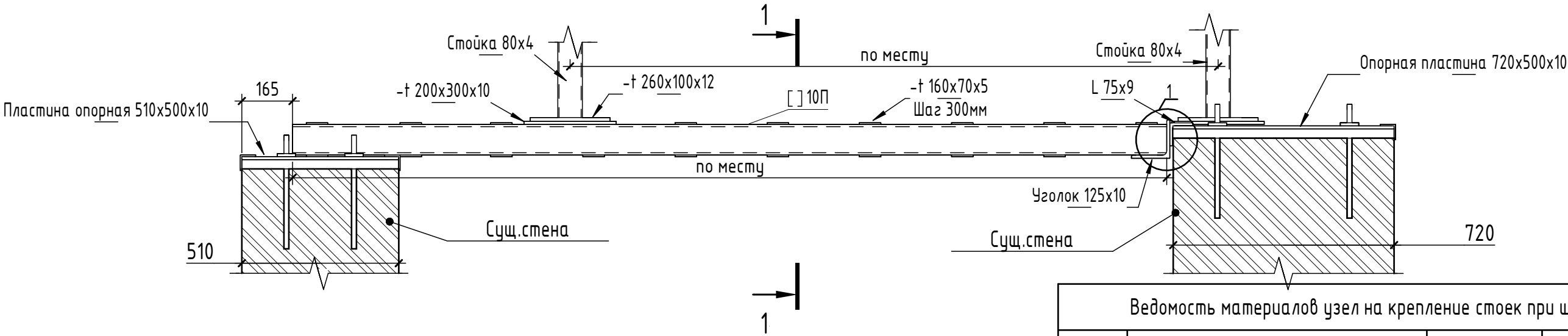
1-1.. (1 : 5)
