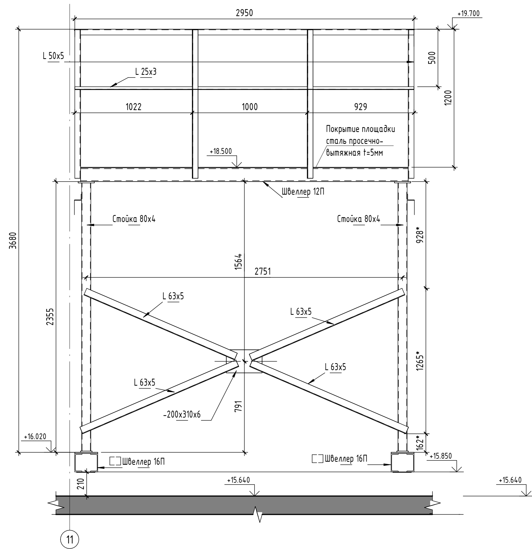
Вид 1 ( 1 : 20)
