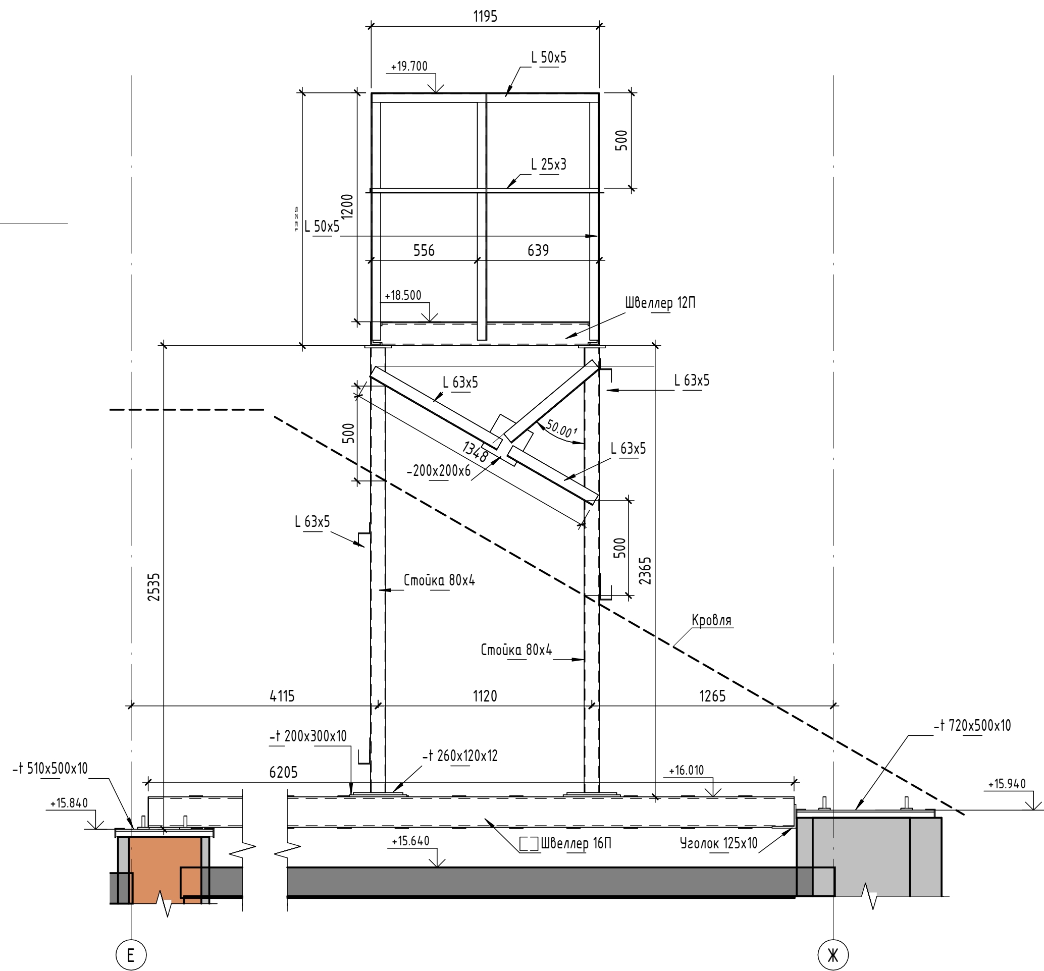
Вид 3 ( 1 : 20)
